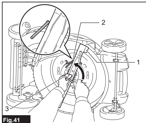
► 1. Cuchilla de la cortadora de césped 2. Pasador 3. Llave de bujías
