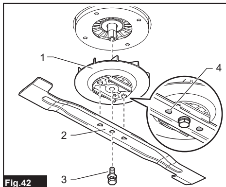
► 1. Soporte de la cuchilla 2. Cuchilla de la cortadora de césped 3. Perno 4. Protuberancia
